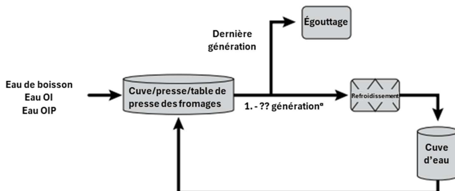
Figure 14: Schéma illustrant la recirculation de l'eau utilisée pour le refroidissement des fromages
