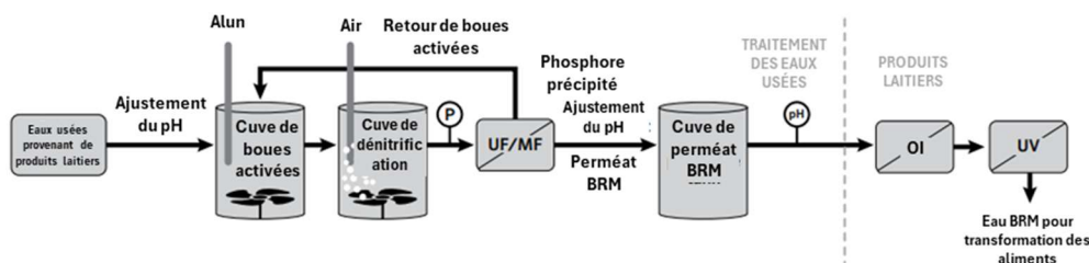
Figure 47: Exemple de récupération de l'eau provenant des eaux de laiterie au moyen d'un BRM et de l'OI
