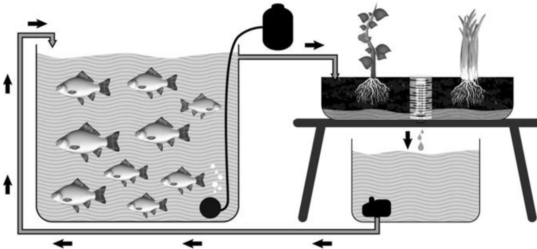
Figure 14. Schéma d'une unité aquaponique simple 4
