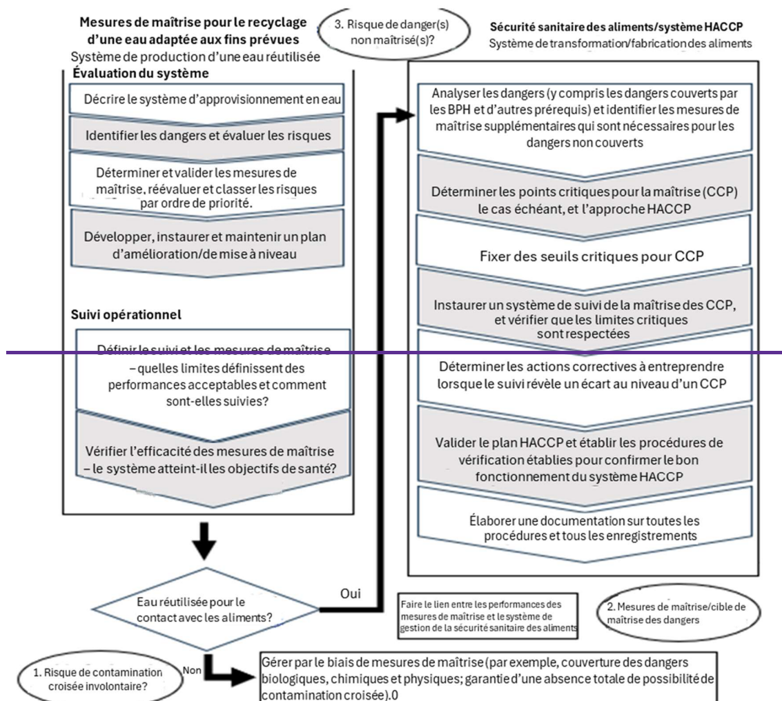
12. Figure 3: Intégration des mesures de maîtrise pour le recyclage de l'eau adaptée aux fins prévues dans le système de sécurité sanitaire des aliments/HACCP (Source: adapté de la publication MRA n° 40, Figure 2).
