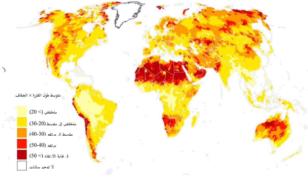
الشكل 3 - درجات شدة حالات الجفاف، 2008 - 1901
