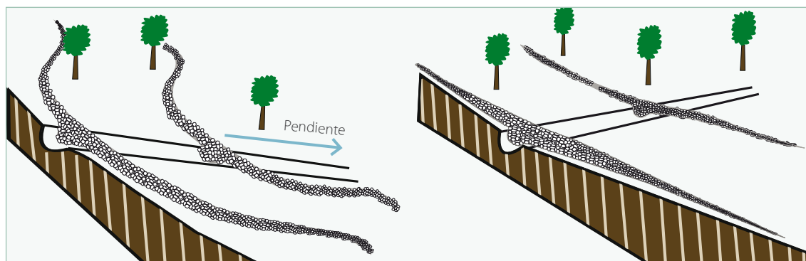
FIGURA 13-VI: Conformación en el terreno de presas permeables de piedras, con bordos de piedra laterales, en nivel y paralelos. Adaptado de Critchley y Siegert (1996).
