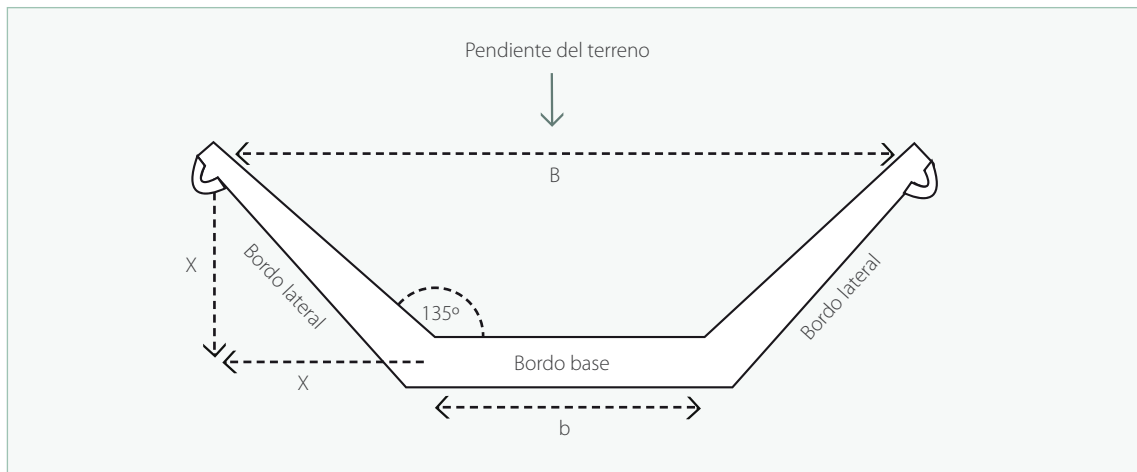
FIGURA 13-I: Configuración de un bordo trapezoidal en el terreno. Adaptado de Critchley y Siegert (1996).
