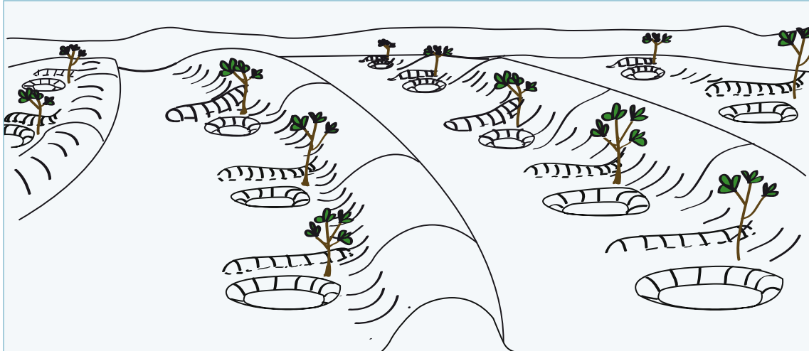
FIGURA 12-XIV: Esquema de cultivos de árboles en surcos y camellones en contorno interceptados (Critchley y Siegert, 1996).
