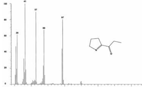
1605 2-Propionylpyrroline (NMR)
