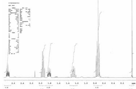
1605 2-Propionylpyrroline (NMR)
