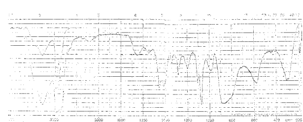
1609 Pyrrolidine (IR)
