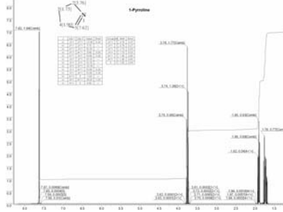
1604 2-Acetyl-1-pyrroline
