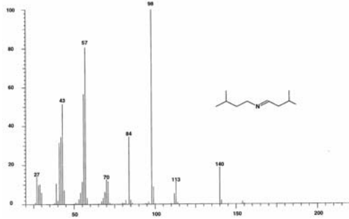
1607 Piperidine
