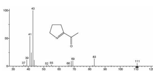
1604 2-Acetyl-1-pyrroline
