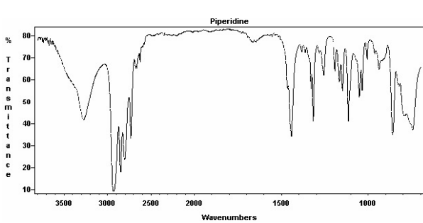
1607 Piperidine
