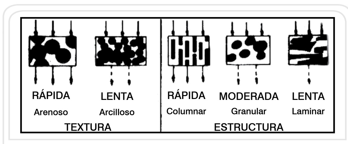
Figura 2. La permeabilidad del suelo en función de la textura y la estructura
