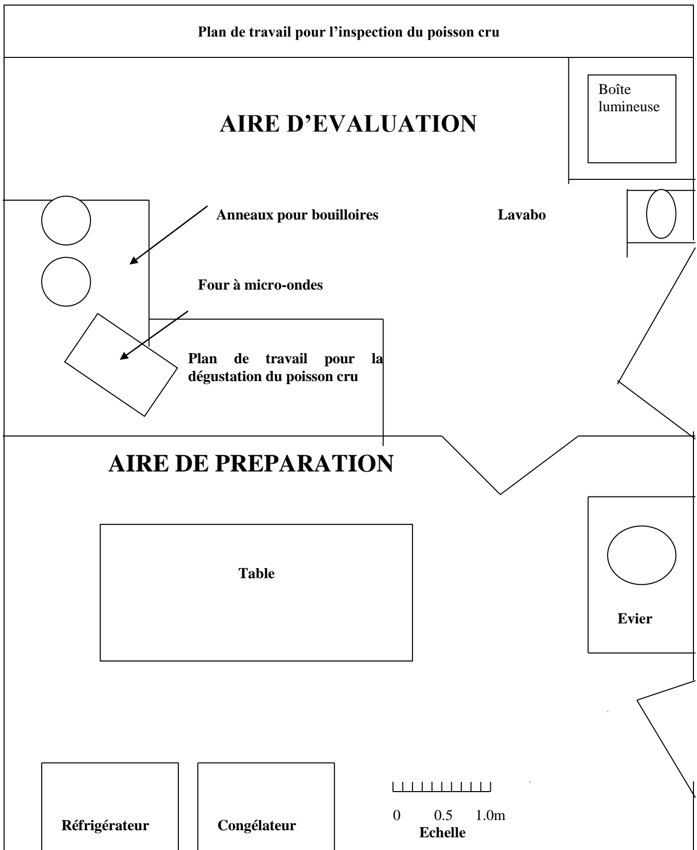
Figure 1. Exemple de plan d'un laboratoire pour l'évaluation organoleptique des produits de la pêche
